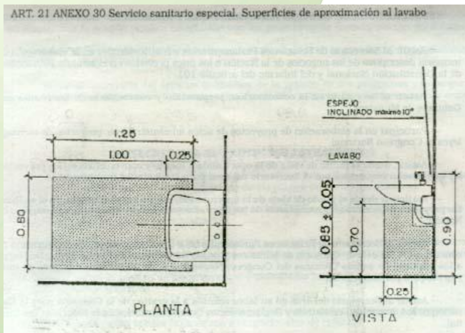
ART. 21 ANEXO 30 Servicio sanitario especial. Superficies de aproximación al lavabo
