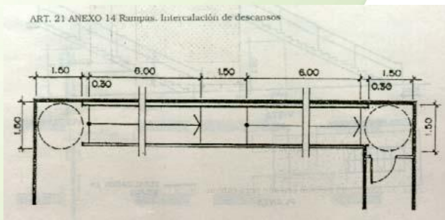
ART. 21 ANEXO 14 Rampas. Intercalación de descansos
