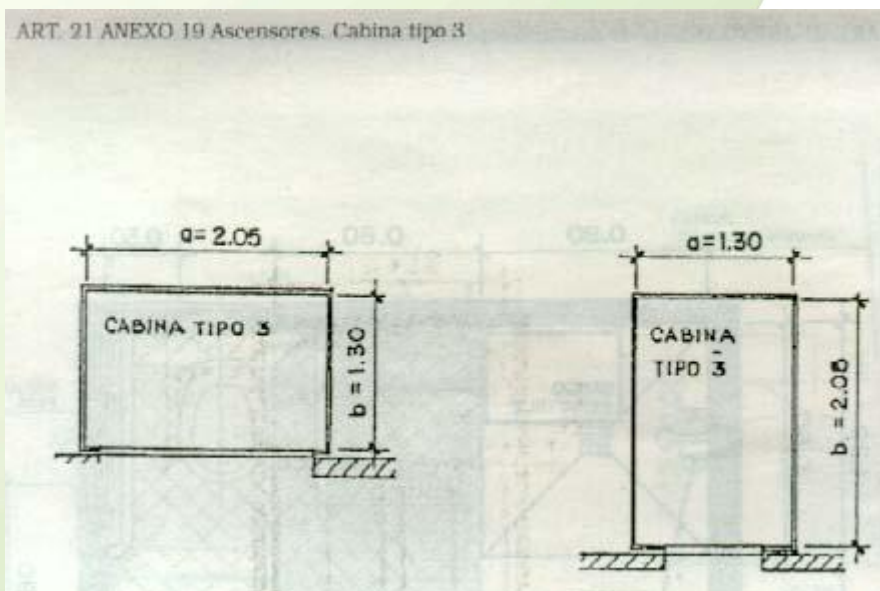
ART. 21 ANEXO 19 Ascensores. Cabina tipo 3
