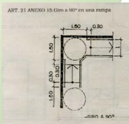
ART. 21 ANEXO 15 Giro a 90° en una rampa
