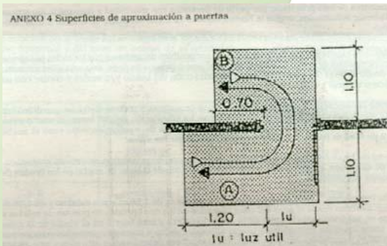
ANEXO 4 Superficies de aproximación a puertas
