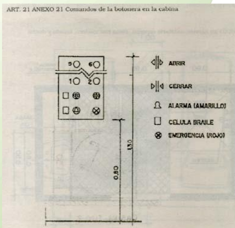
ART. 21 ANEXO 21 Comandos de la botonera en la cabina
