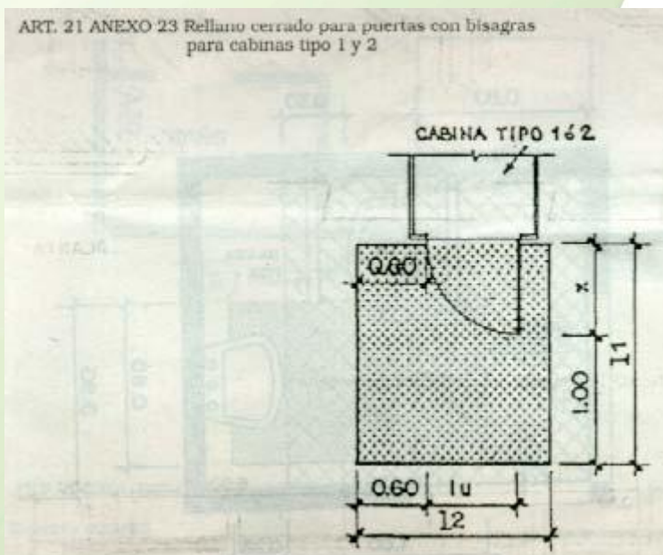
ART. 21 ANEXO 23 Rellano cerrado para puertas con bisagras para cabinas tipo 1 y 2
