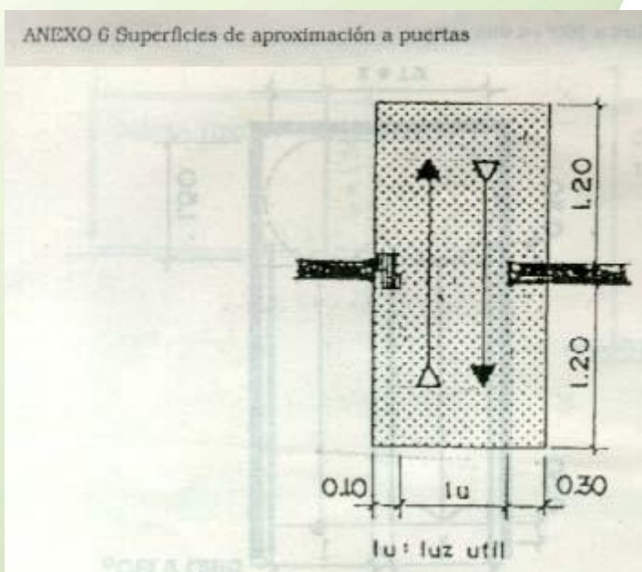
ANEXO 6 Superficies de aproximación a puerta
